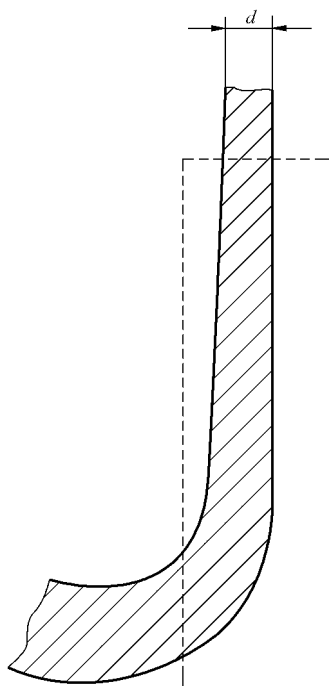
图 B.1 筒体/瓶底过渡区
