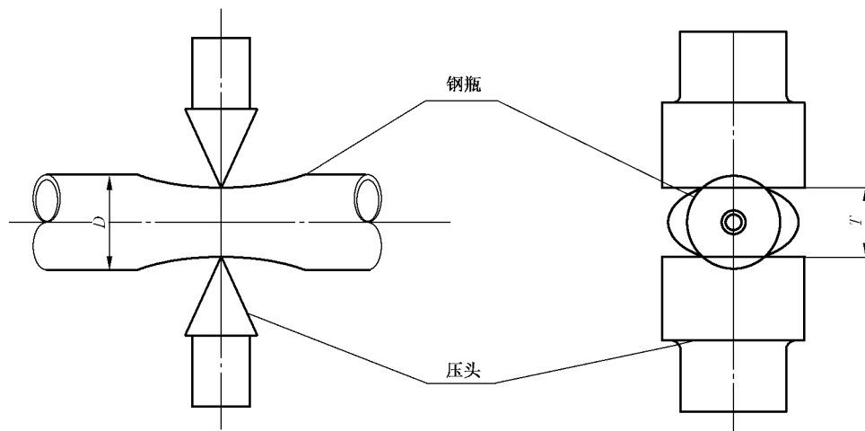
图 D.3 压扁试验示意图
