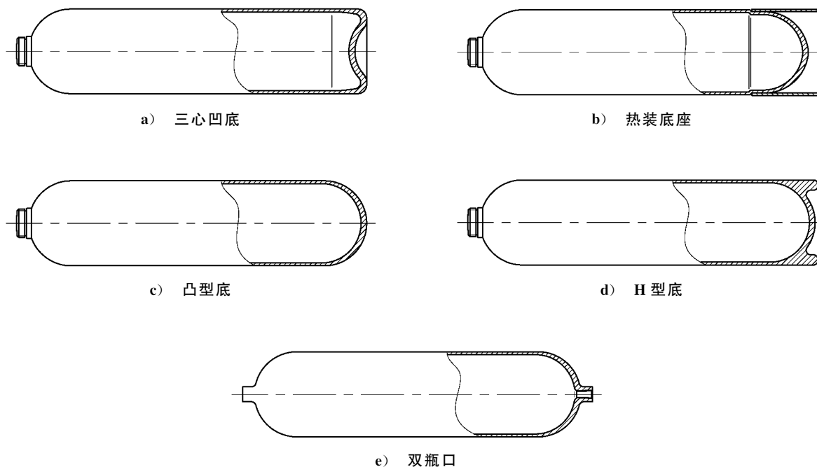
图 1 结构型式
