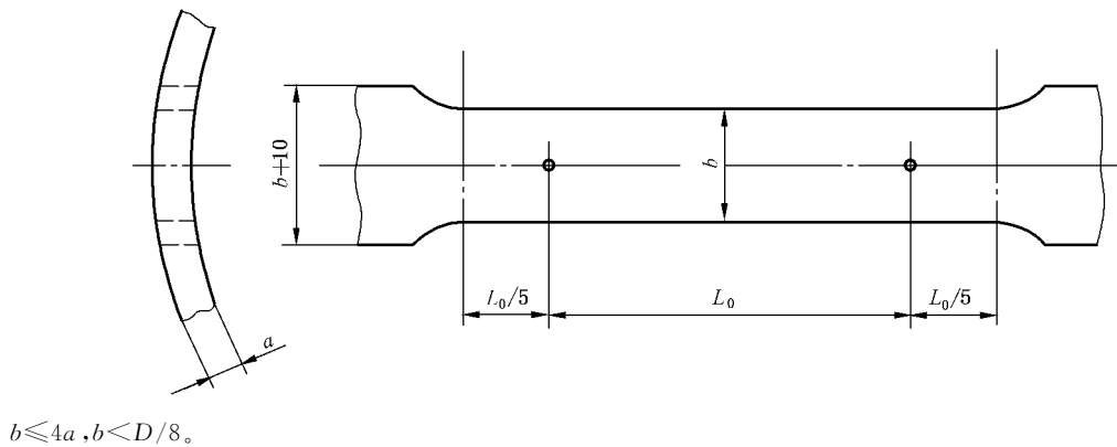
图 5 拉伸试样图
