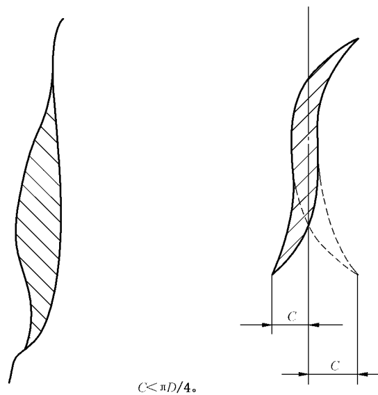
图 10 破口形状尺寸示意图
