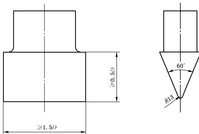
图 D.2 压头的形状尺寸
